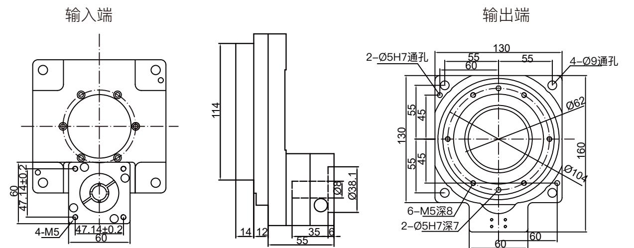
步进电机 / Stepping Motor
