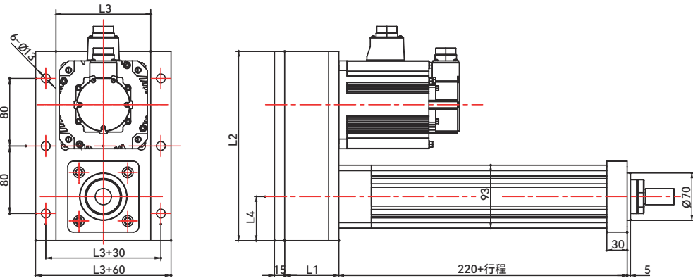
M6:尾部法兰
