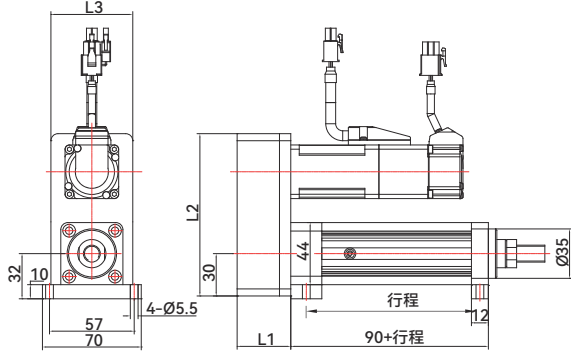
M2:卧式底座
