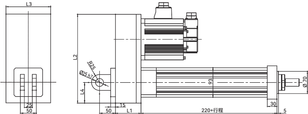
M4:尾部双耳轴
