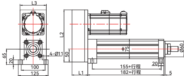
M2:卧式底座
